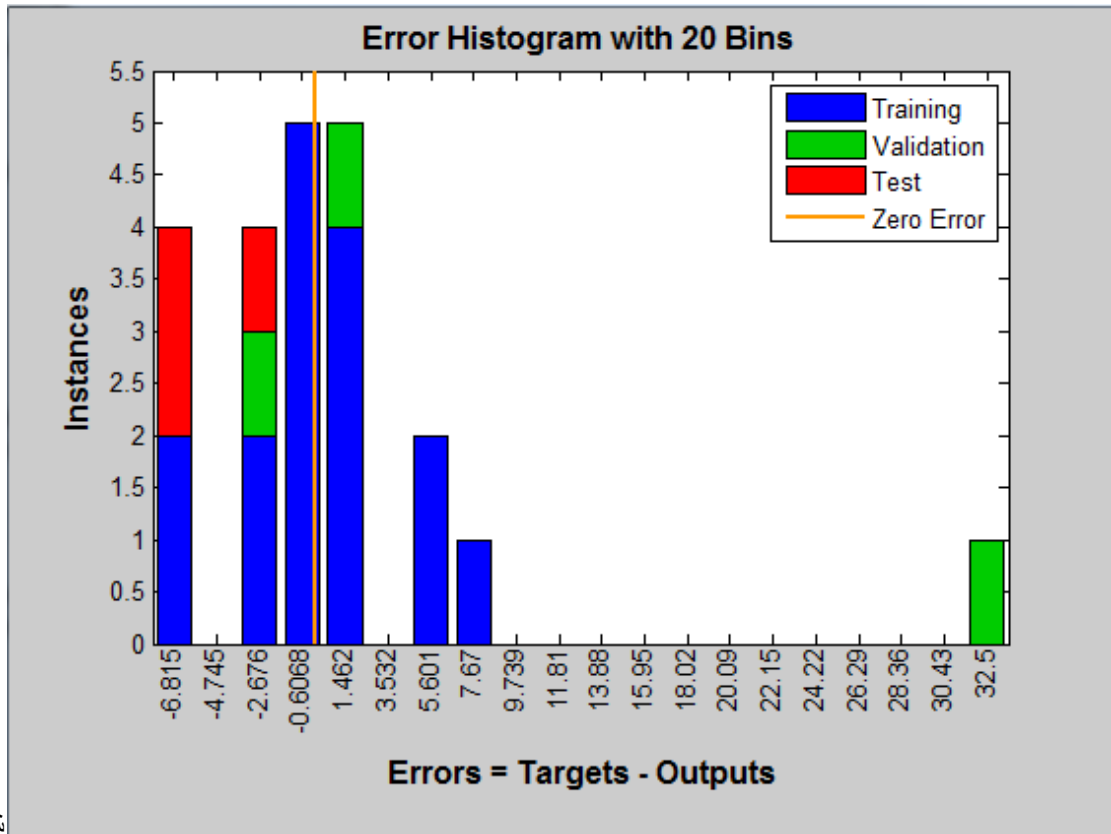
رقم ( ٦ ) يبين مدرج الأخطاء
