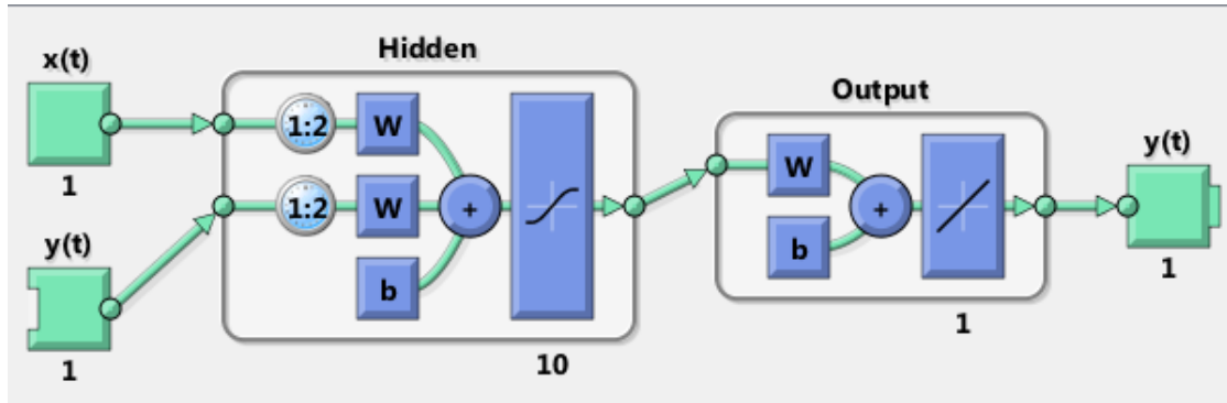
شكل رقم ( ٤ ) البنية المعمارية للشبكة العصبية
