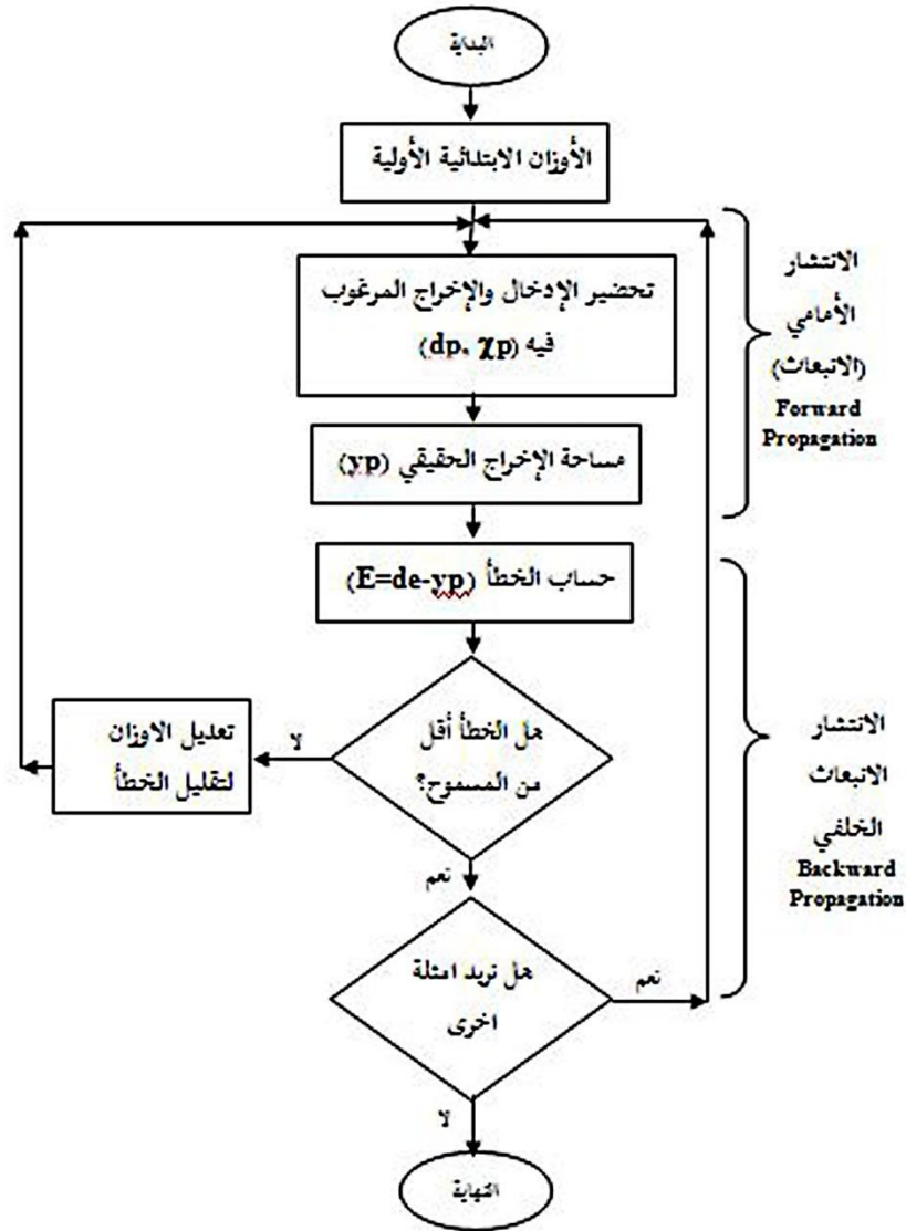
شكل ( ٣ ) خوارزمية الانبعاث الخلفي ( back propagation )
