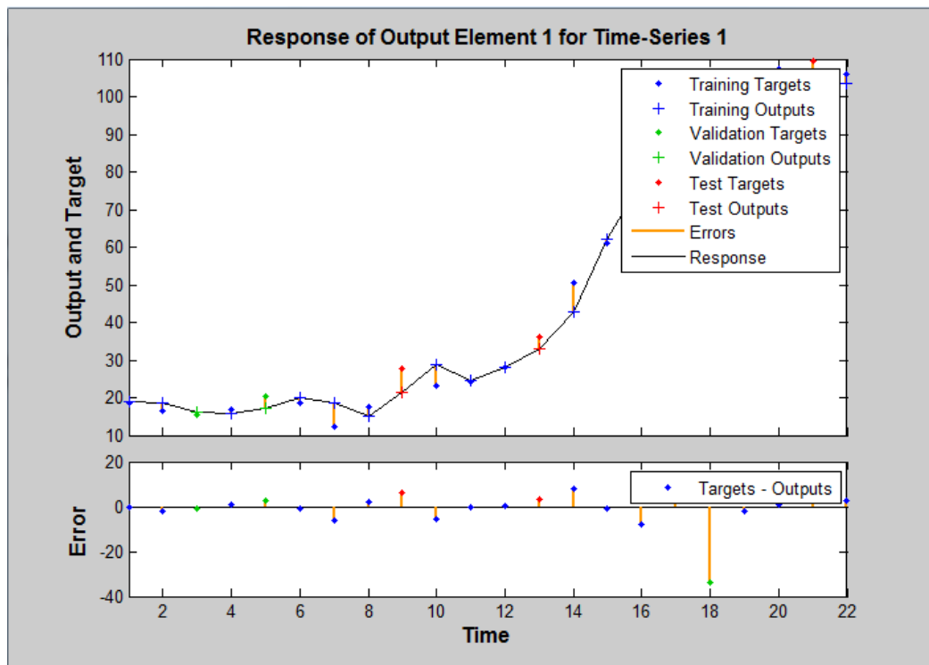
شكل رقم ( ٧ ) يبين استجابة السلسلة الزمنية
