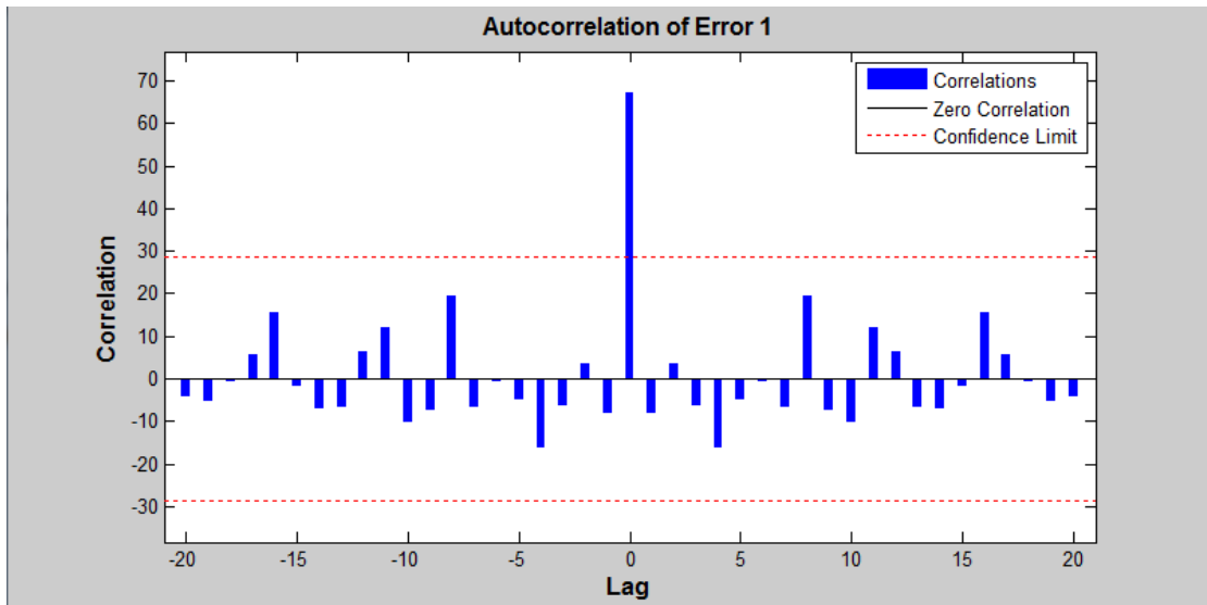
شكل رقم ( ٩ ) يبين الارتباط الذاتي للأخطاء العشوائية
