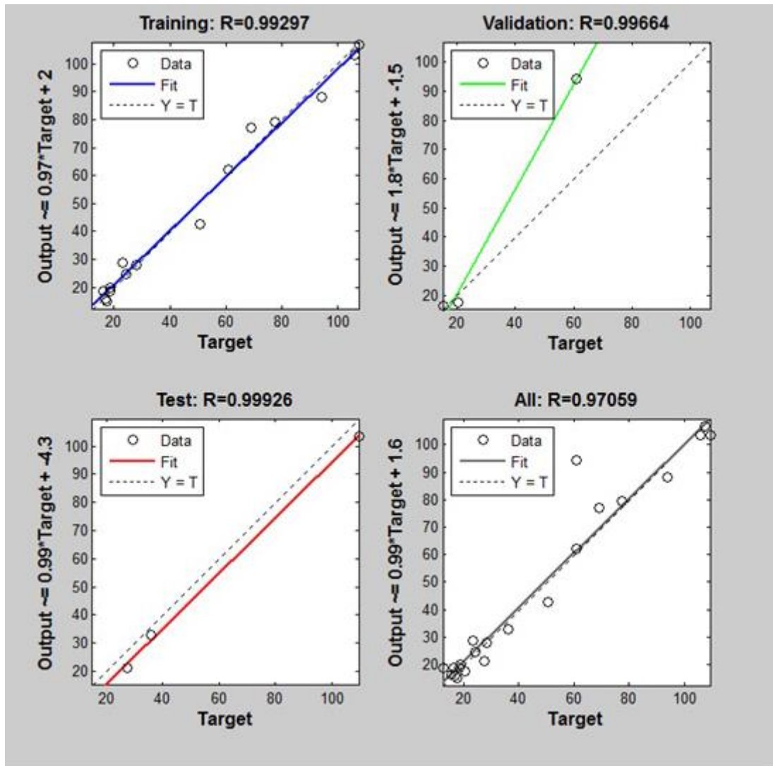
شكل رقم ( ٨ ) يبين معادلة الانحدار
