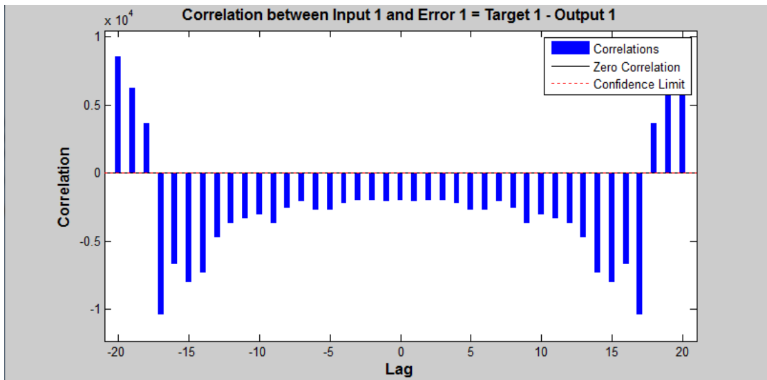
شكل رقم ( ١٠ ) يبين الارتباط بين المدخلات و الأخطاء العشوائية
